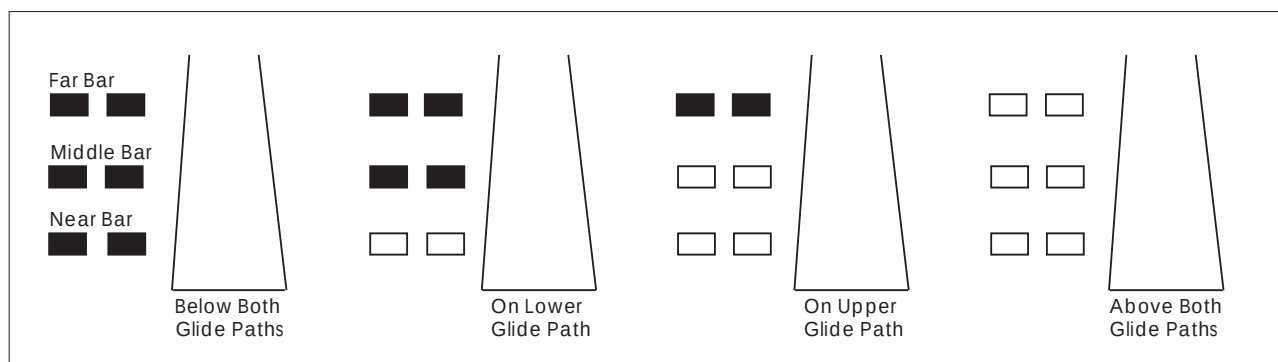
FIG 2-1-3 3-Bar VASI
